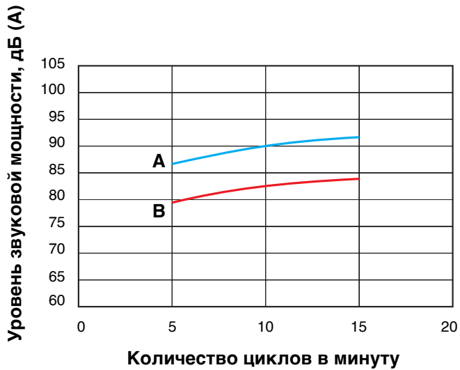
Звуковая мощность N22DN0
