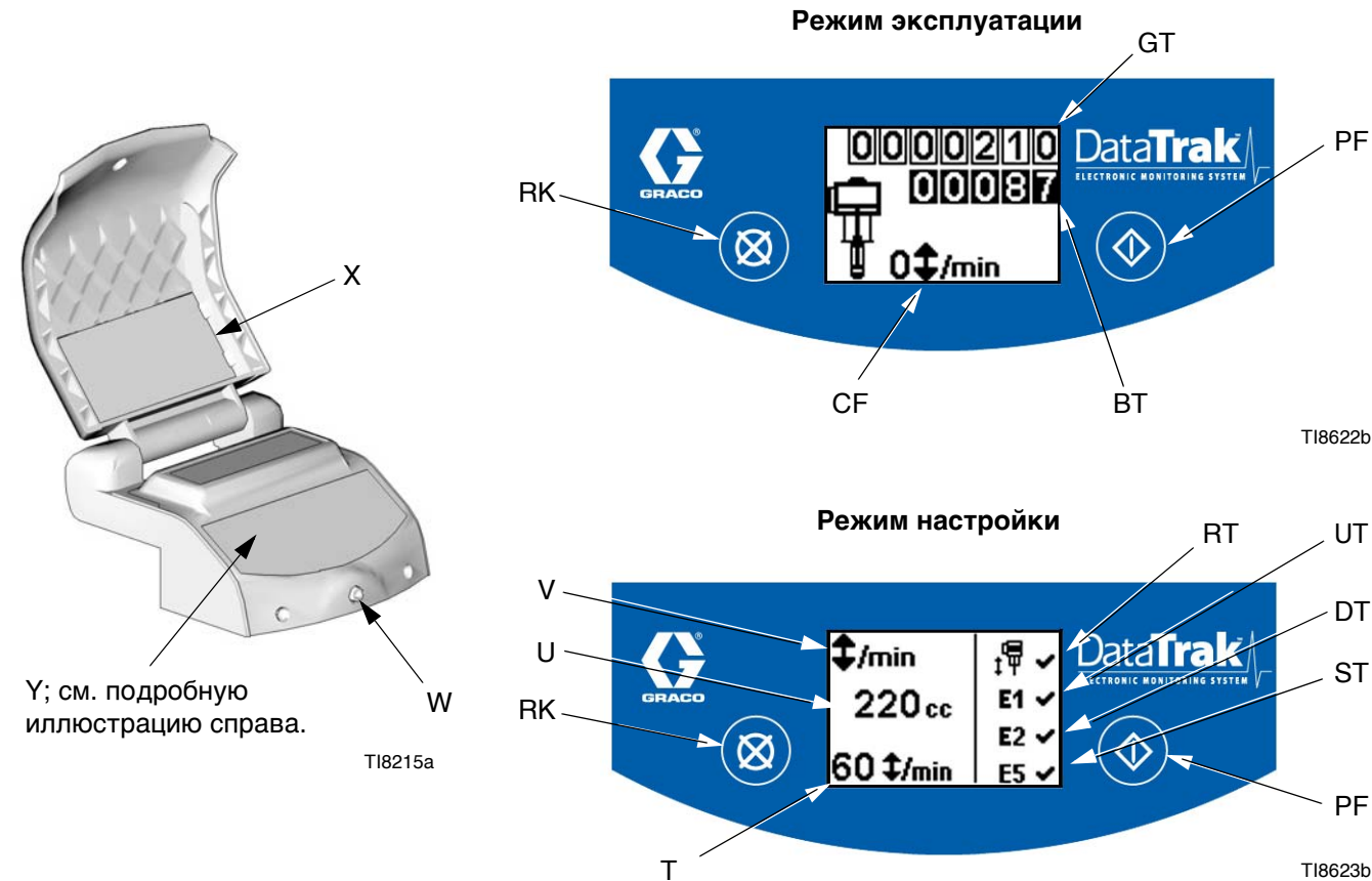
Рис. 3. Устройства управления модулем DataTrak и их индикаторы
