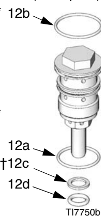
Узел тарелки (12) (см. стр. 25)
