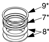
Порядок установки уплотнений
