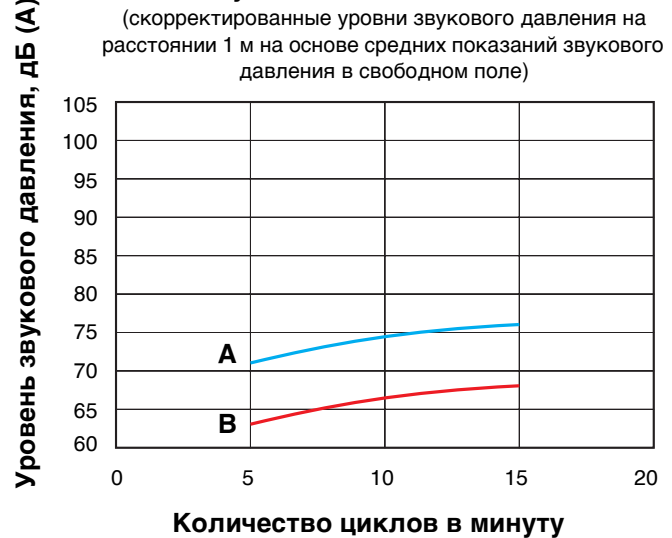
Звуковое давление N22LN0
