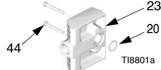
Узел дистанционного выхлопного устройства (23)
