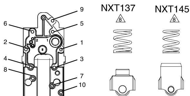
Врезка 11a. Порядок затягивания винтов
