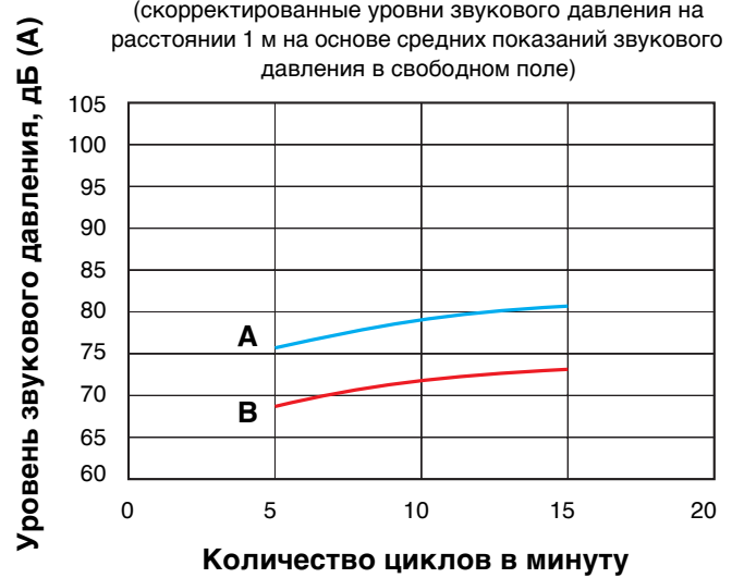
Звуковое давление N22DN0
