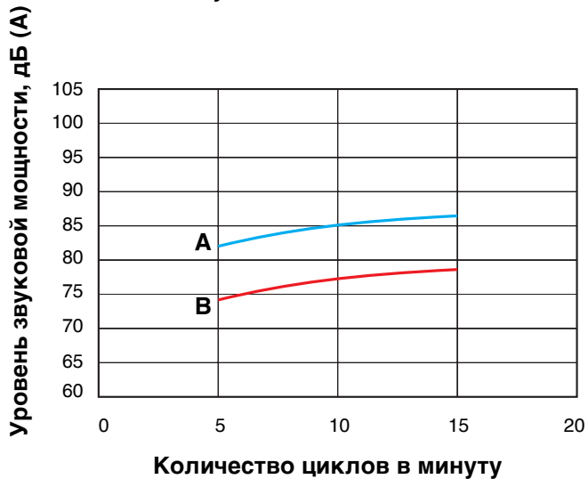
Звуковая мощность N22LN0
